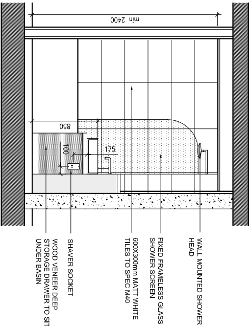
ELEVATION B
