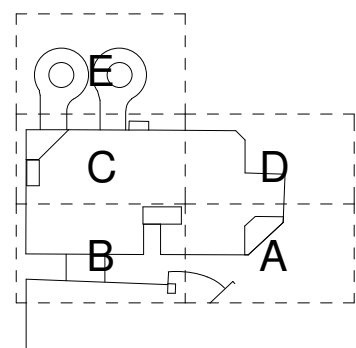
01 DOOR TYPE 201 - Single Door Set SCALE 1:20
