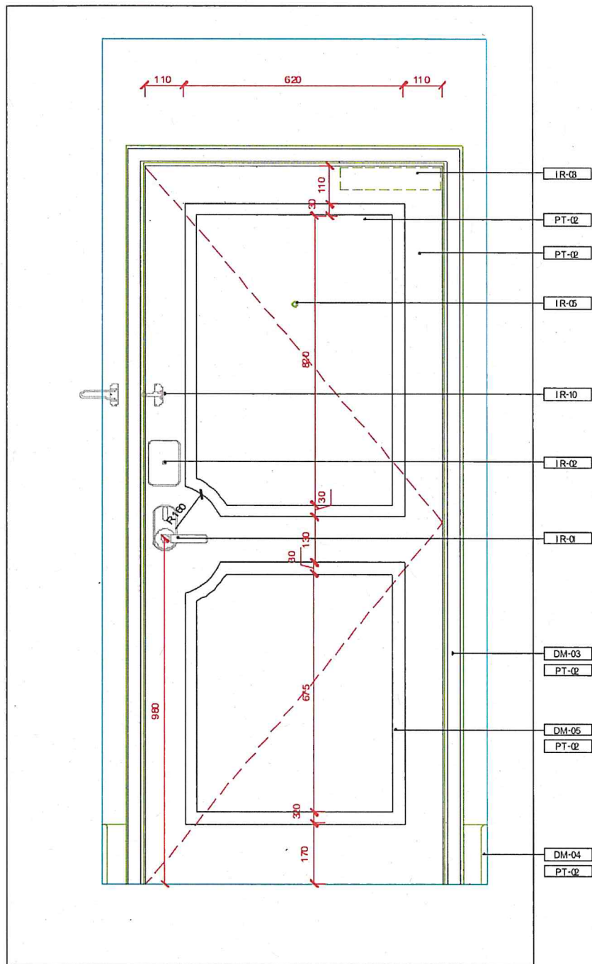
E1 | ELEVATION 01 - BEDROOM SIDE SCALE 1:10
